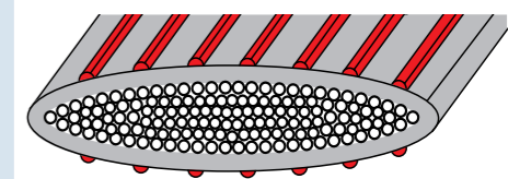
Renforcement nervuré amélioré
