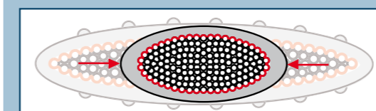
Sezione sotto carico (WLL) a confronto
