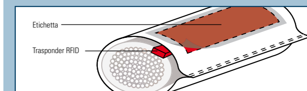
Etichetta protetta con trasponder RFID
